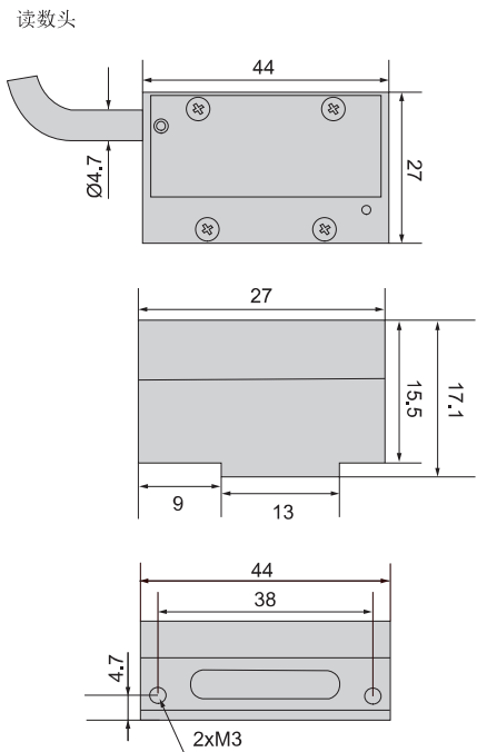
钢带光栅尺
